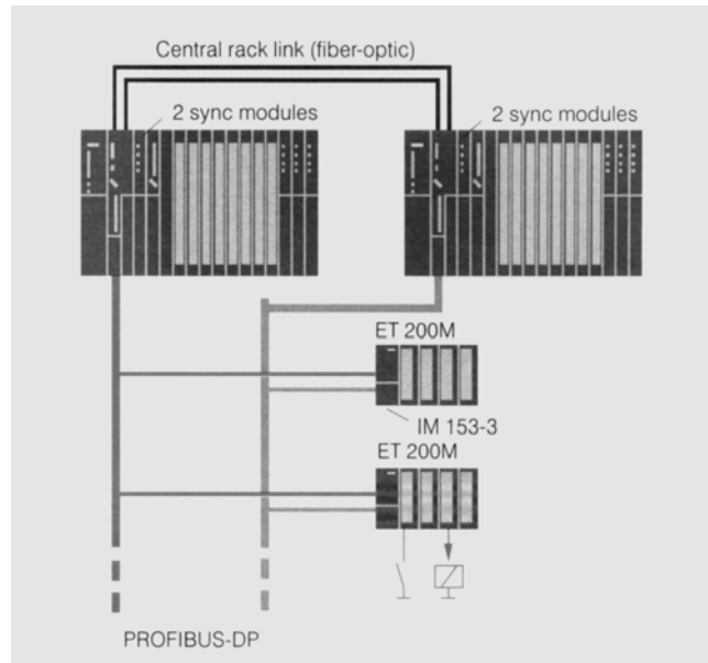
图 10 切换式配置
